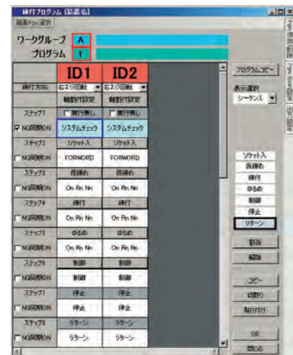
MU50 締付プログラム設定画面
